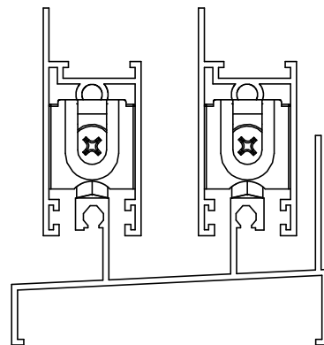
DETALHE DA MONTAGEM (SEM ESCALA)
