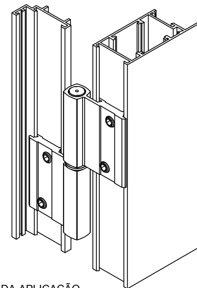
DETALHE DA APLICAÇÃO (SEM ESCALA)
